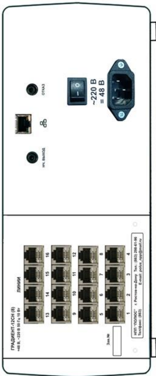
Рис. 2.2. Внешний вид 16-ти канального регистратора со стороны задней панели
